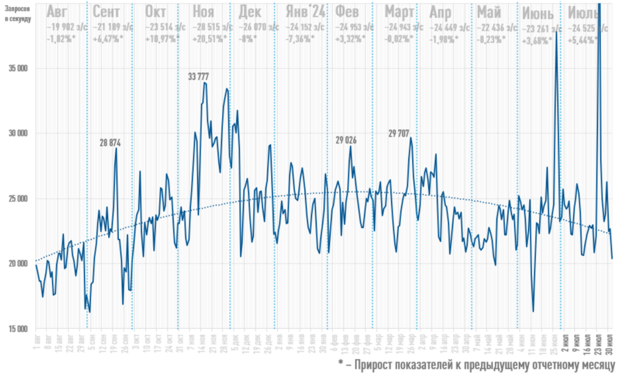
График запросов в секунду к корневым серверам
